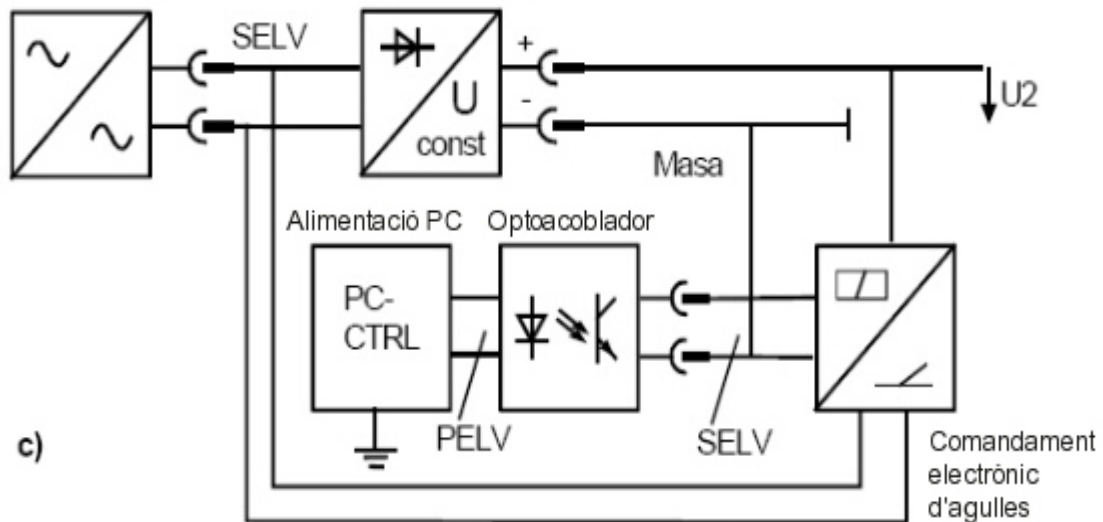
Comandament electrònic d'agulles
