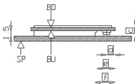
Descodificador, vista lateral
