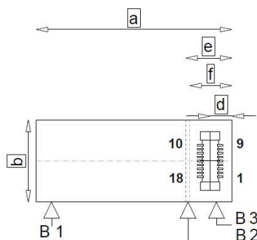
Vista desde debajo, lado componentes del soporte
