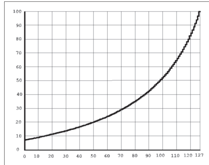
Característica de velocidad máxima (ver CV05/par013) en velocidad de maniobras (ver CV61 / par018)
